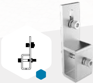
TZ001 - Suporte Metálico Zipado Telha Zipada - Alumínio e Inox Telhas Metálicas Zipadas
