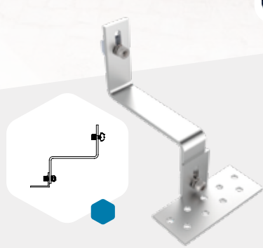
TC002 - Suporte Metálico Gancho em Alumínio / Inox - Telhas Ceramicas / Concreto / Modelo Capa Canoa e outros
