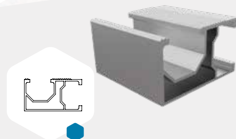
H2 2200 - Perfil ALH2 Perfil ALH2 - 50 X 30 mm Comprimento 2200 mm
