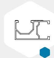
H2 2200 - Perfil ALH2 Perfil ALH2 - 50 X 30 mm Comprimento 2200 mm
