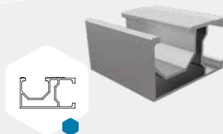
H2 2200 - Perfil ALH2 Perfil ALH2 - 50 X 30 mm Comprimento 2200 mm
