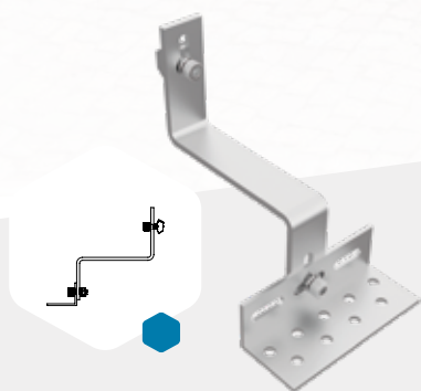
TC001 - Suporte Metálico Gancho em Alumínio / Inox - Telhas Ceramicas / Concreto / Todos Modelos
