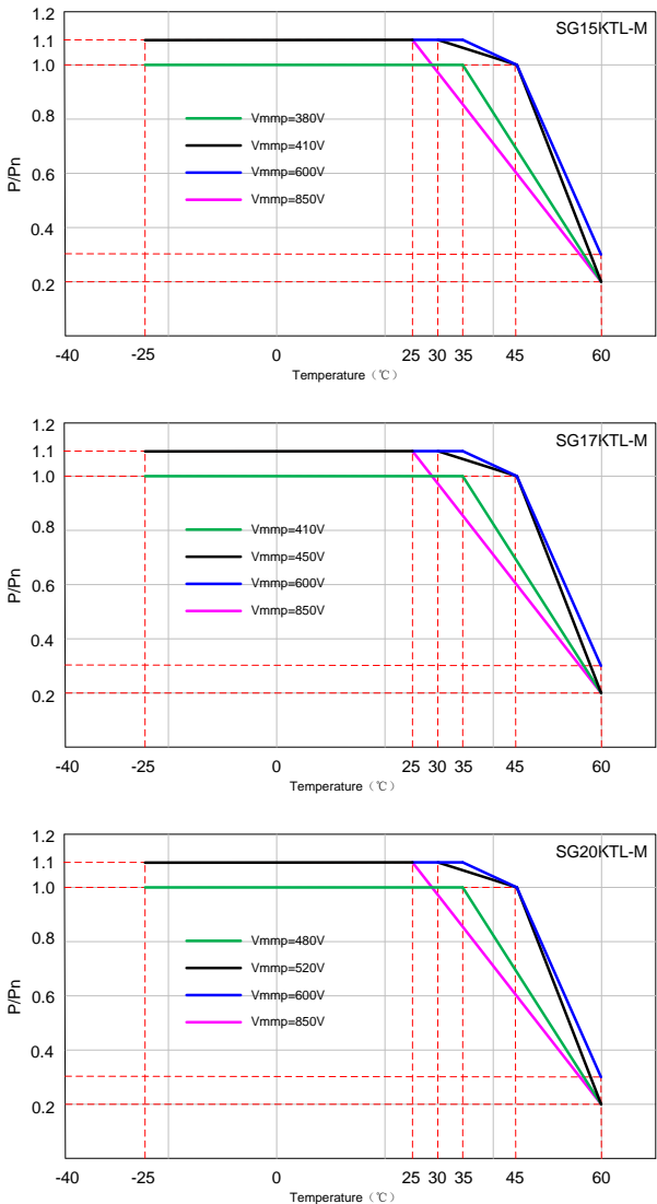
Fig. 2-6 Desclassificação por sobretemperatura(Pf=1)
