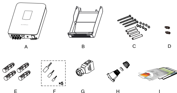
Fig. 4-4 Escopo da Entrega
