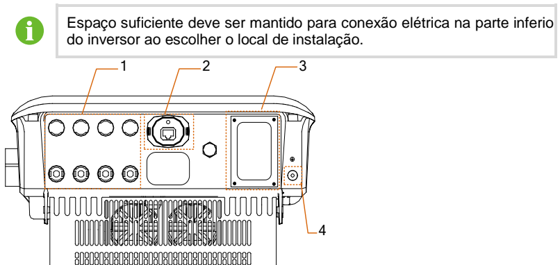
Fig. 6-1 Área de conexão de cabos
