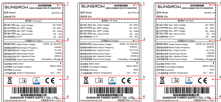
Fig. 4-2 Placa de identificação dos inversores
