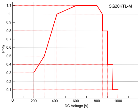
Fig. 2-8 Tensão de entrada e desclassificação de potência(Pf=1)
