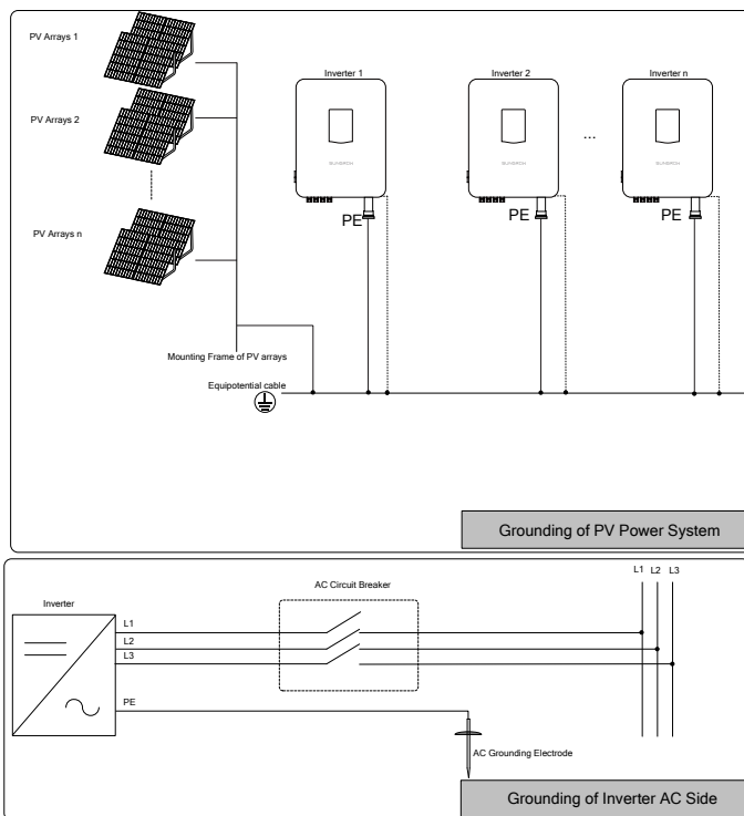
Fig. 6-2 Aterramento do Inversor
