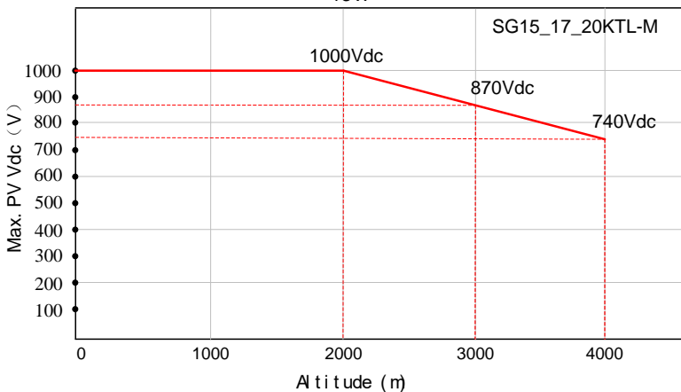
Fig. 2-9 Curva de desclassificação por altitude
