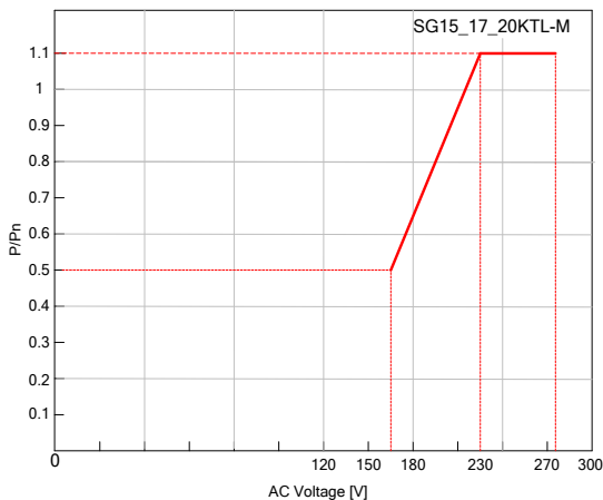
Fig. 2-7 Desclassificação por subtensão(Pf=1)
