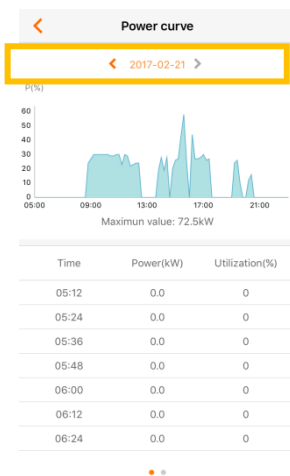
Fig. 10-12 Curva de potência
