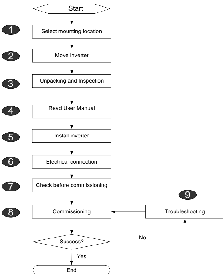
Fig. 3-1 Fluxograma de instalação
