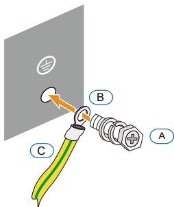
Fig. 6-4 Conexão do Segundo PE
