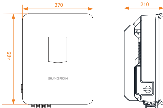
Fig. 2-3 Dimensões do inversor (em mm)
