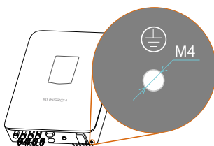
Fig. 6-3 Segundo terminal PE
