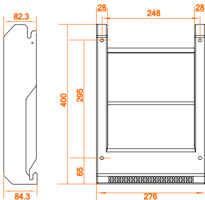
Fig. 5-1 Dimensões da placa traseira (dimensões em mm)
